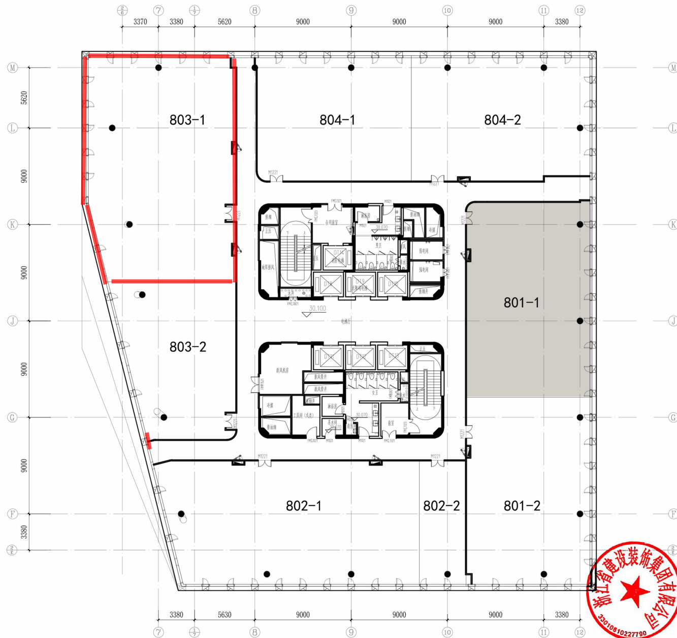
八层平面
