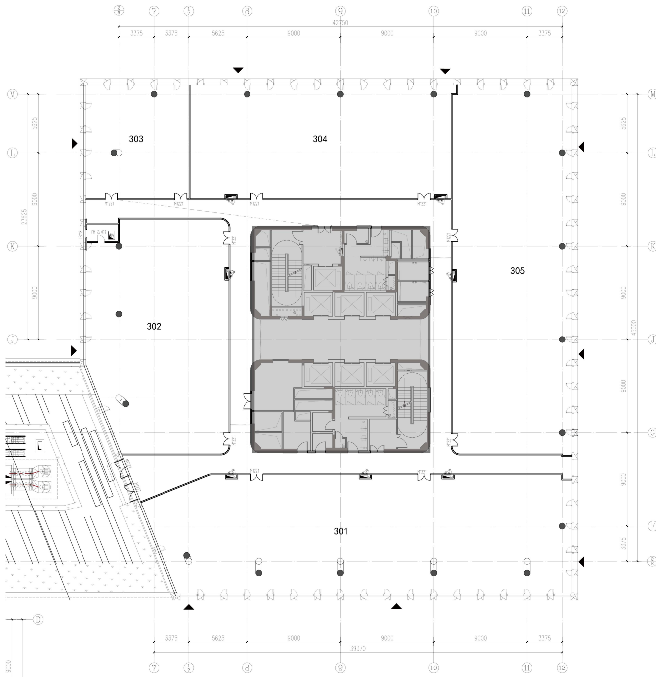
三层平面图局部图
