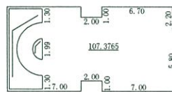
二层平面图
