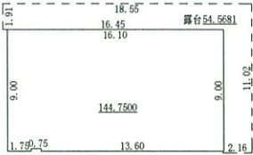
二层平面图 (结构层高: 4.25m)
