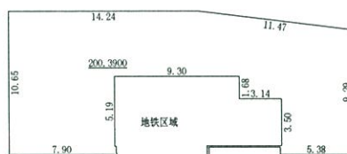
一层平面图
