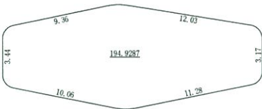
一层平面图
