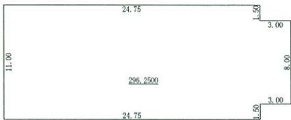
一层平面图 (结构层高: 4.00、4.30、7.75m)
