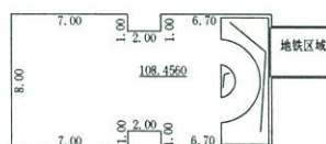
二层平面图
