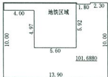
一层平面图
