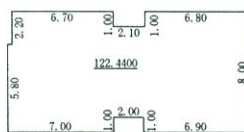
二层平面图
