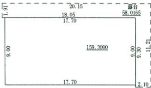
二层平面图
