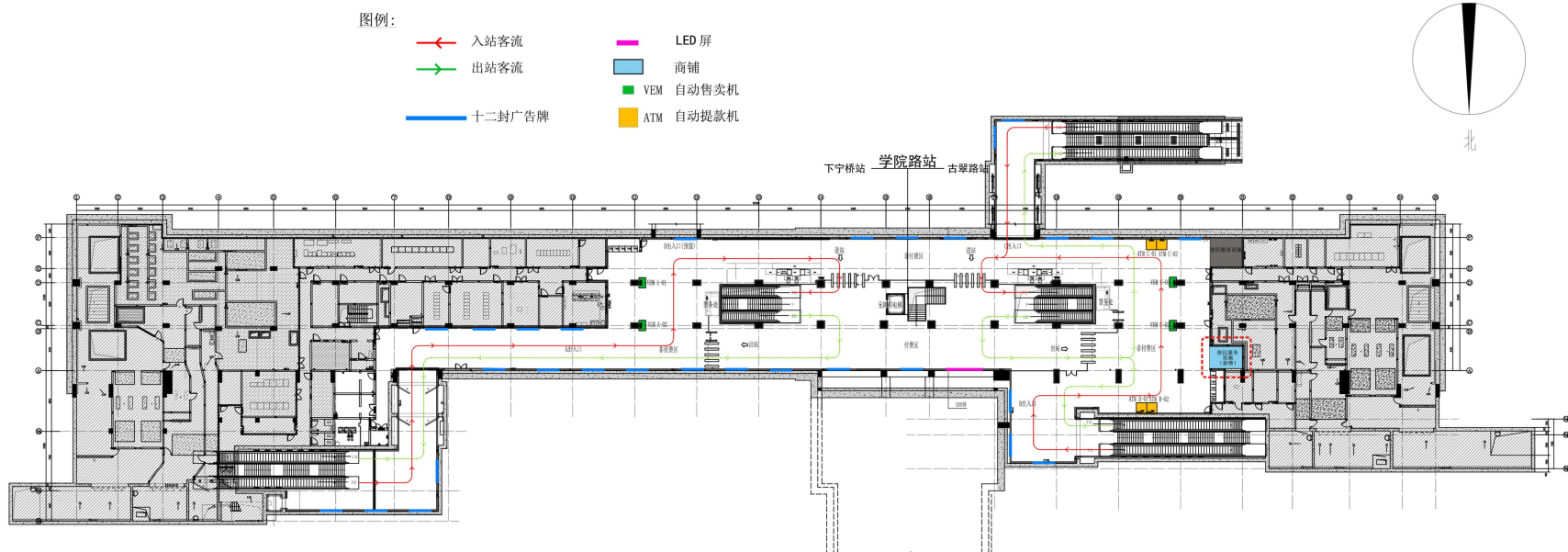
站厅层平面布置图
